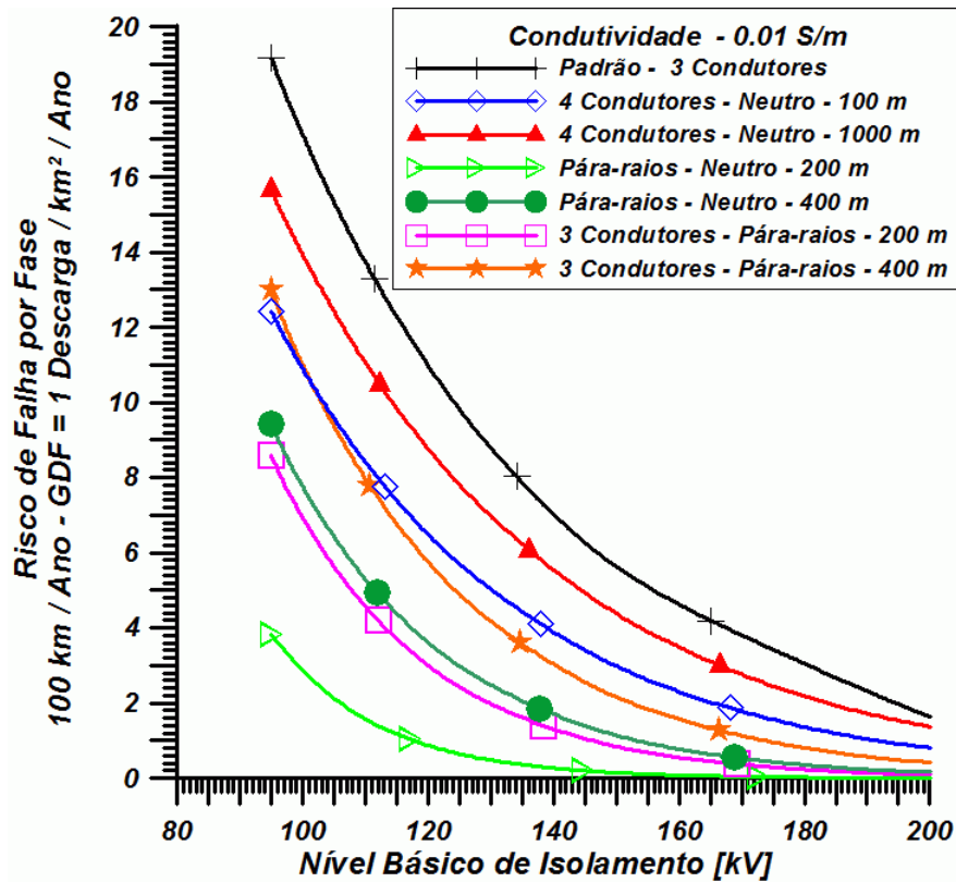
Figura 5 – Risco de Falha para uma Distância de Influência de 20 Postes, Condutividade do Solo = 0,01 S/m e GDF = 1 Descarga ao Solo por km 2 por Ano.
