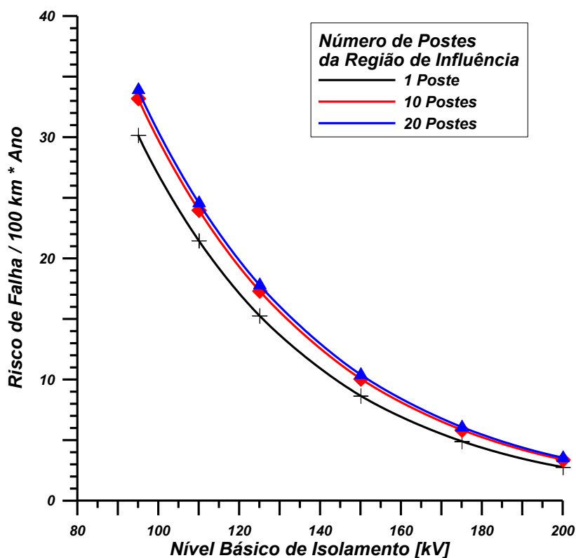
Figura 4 – Risco de Falha por Fase x Nível Básico de Isolamento para uma Linha de Distribuição sem Cabo de Neutro e Pára-raios com Solo de 0.0033 Siemens/metro, para GDF= 1 Descarga ao Solo por km 2 por Ano.
