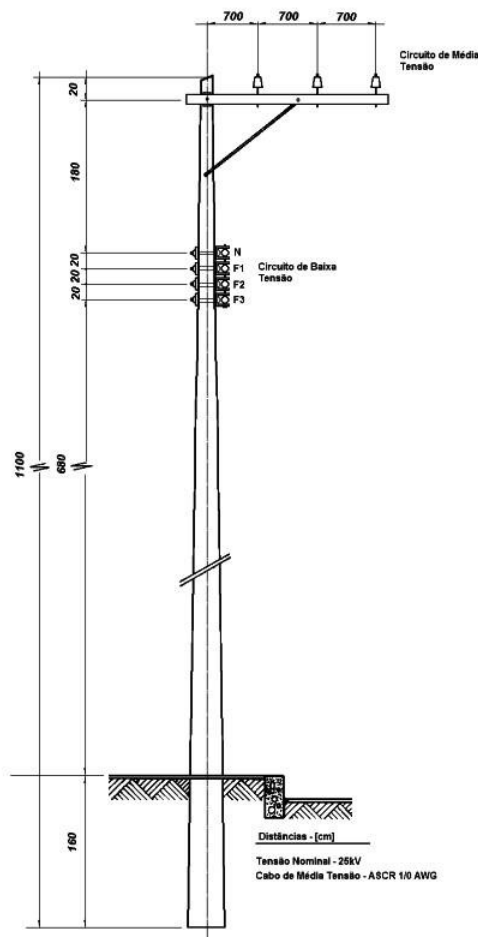
Figura 2 – Geometria dos condutores da linha aérea considerada.
